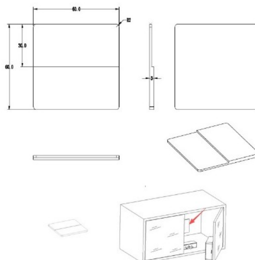
Double Door Striker
